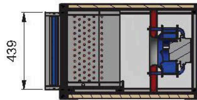
A-A (1:15)
